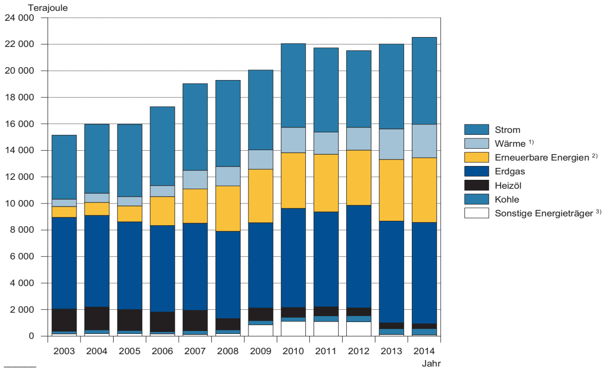
Energieverwendung der Industriebetriebe in Mecklenburg-Vorpommern 2003 bis 2014 nach Energieträgern
