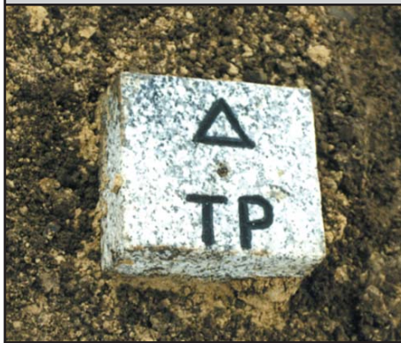
BFP/TP Granitpfeiler 16 cm x 16 cm (auch bodengleich)*
